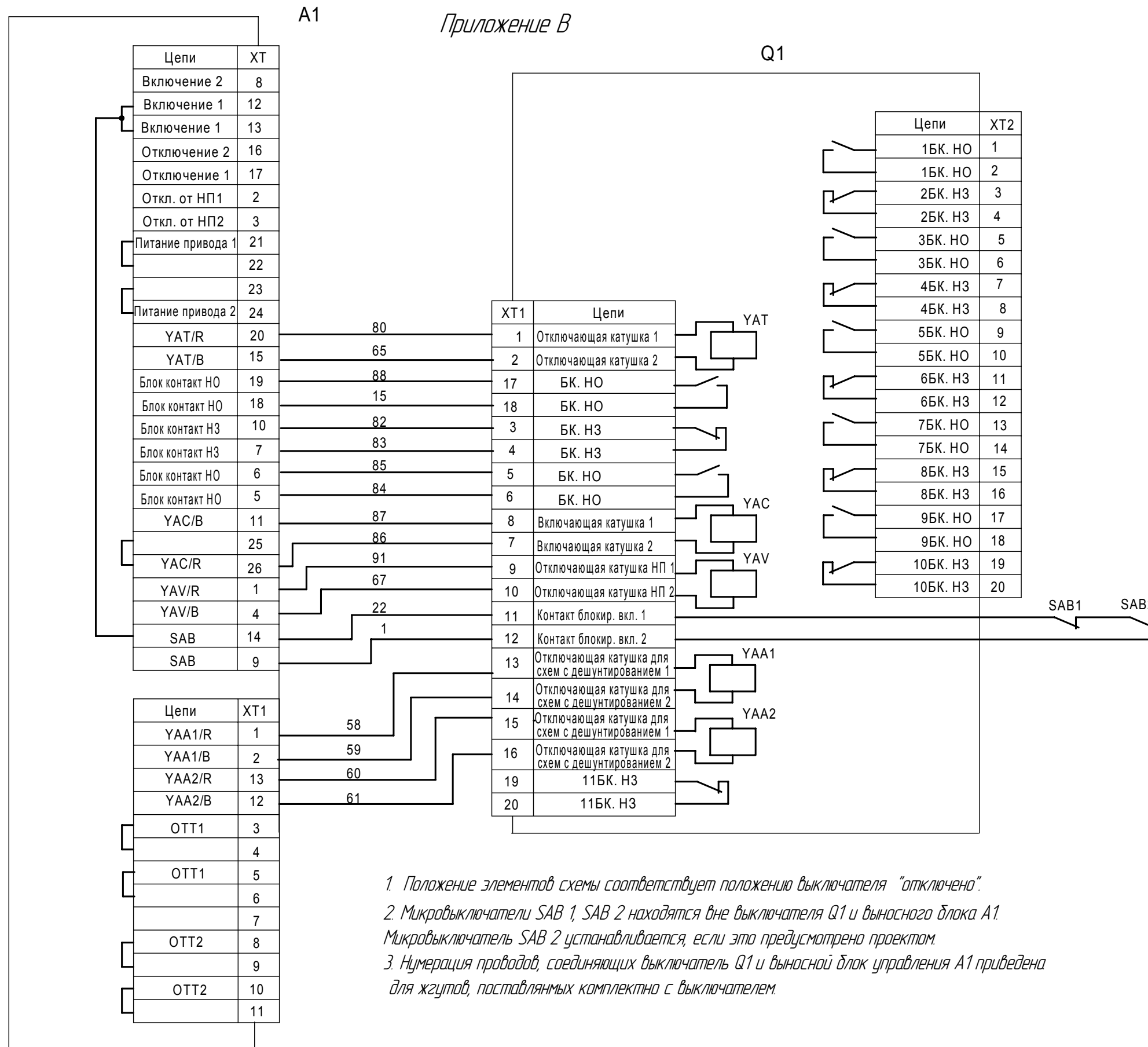
Рисунок В.1 – Вариант 14 – схема электрическая принципиальная выключателей вакуумных серии ВР1 (переменный, постоянный ток 220В; с блокировкой от повторного включения (KBS), с цепью отключения от независимого питания (YAV) и цепями отключения для схем с дешунтированием (YAA1, YAA2))
