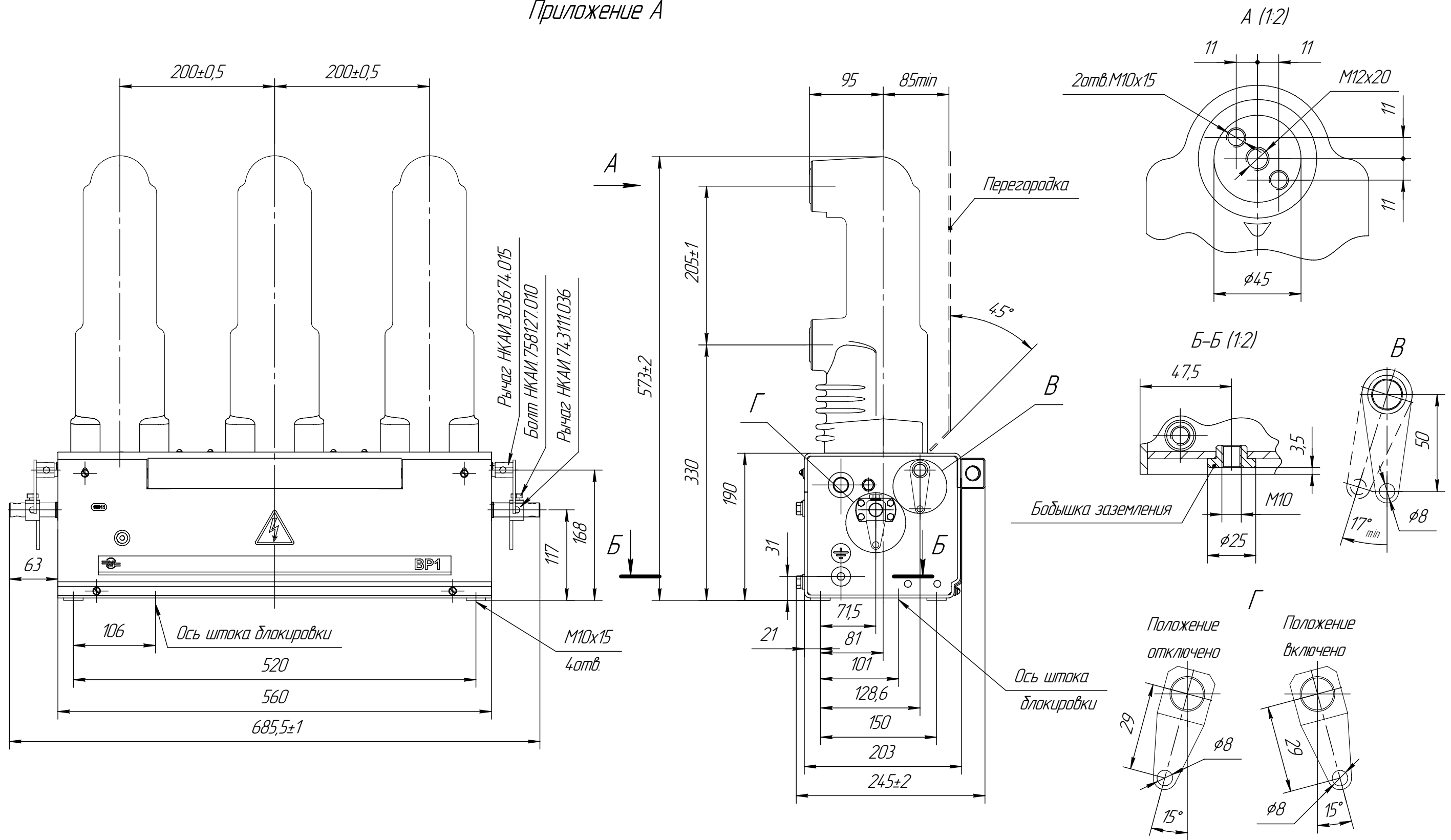
Рисунок А.1 – Габаритные, установочные и присоединительные размеры выключателей вакуумных серии ВР1 с валами отключения с установленными рычагами НКАИ.303674.015 и с валами для блокировки с установленными рычагами НКАИ.743111.036
