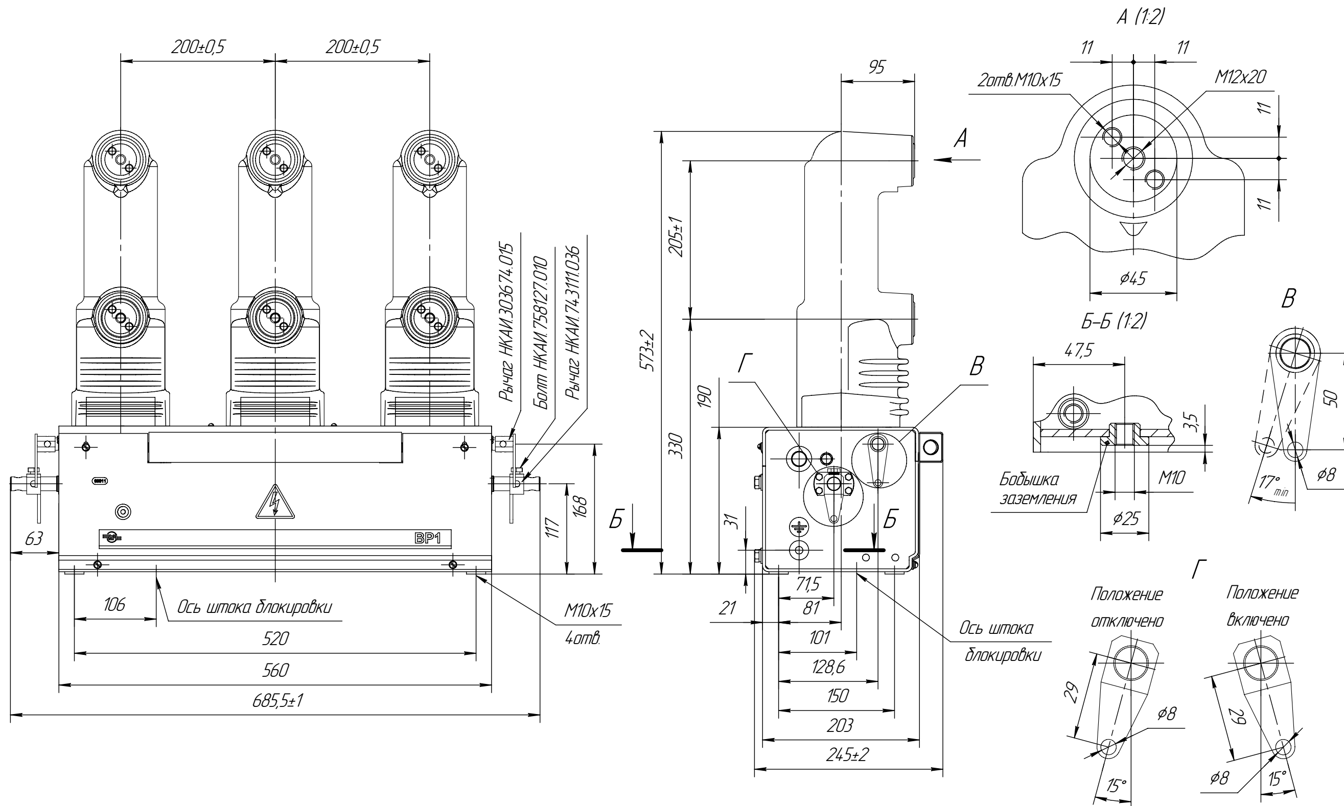
Рисунок А.3 – Габаритные, установочные и присоединительные размеры выключателей вакуумных серии VP1 с валами отключения с установленными рычагами НКАИ.303674.015 и с валами для блокировки с установленными рычагами НКАИ.74.3111.036 с контактами полюсов со стороны клеммных рядов
